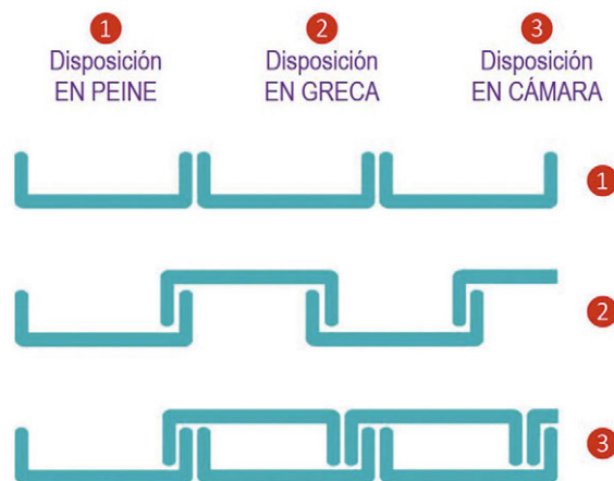
Fig. 4: vista en planta de las tres formas características de disponer los perfiles de vidrio en U.
